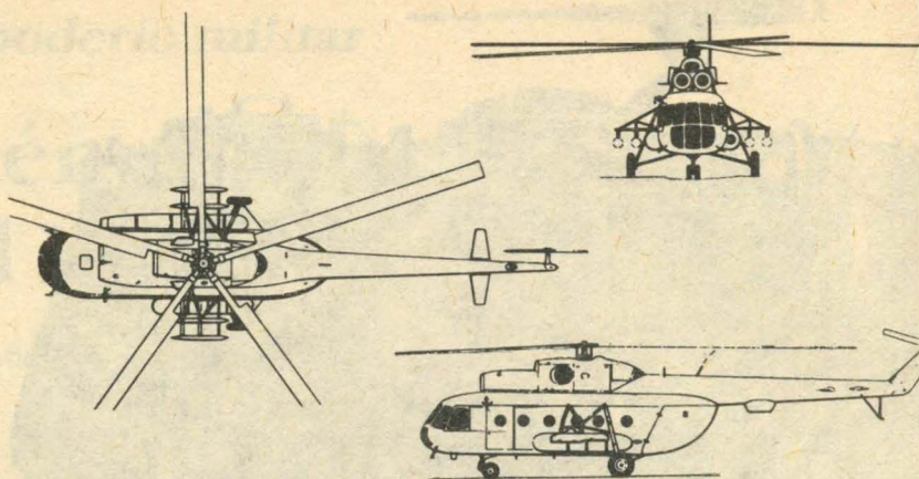
Diagrama del MI 8 (URSS): carga hasta 12 mil kilos.
